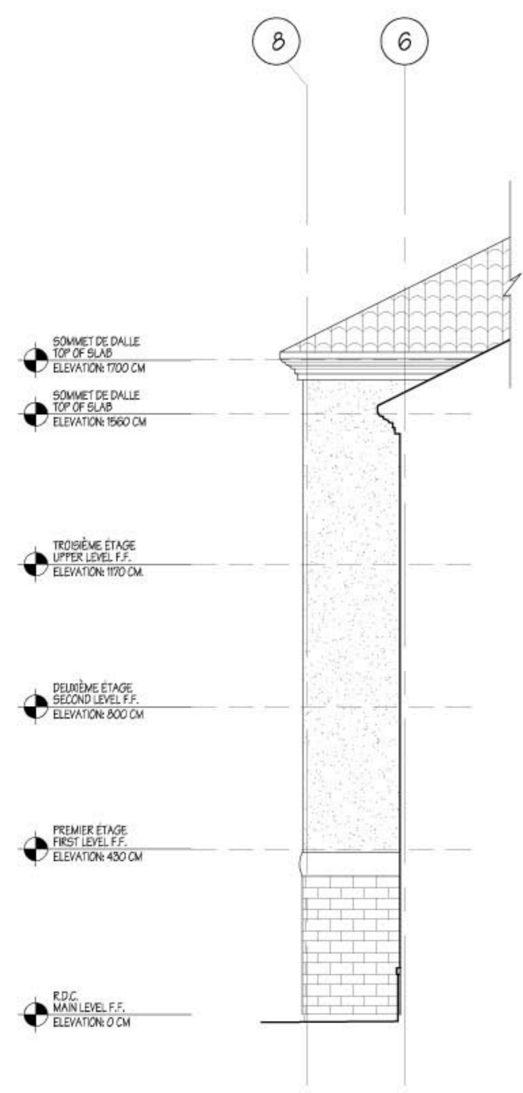
3 ÉLEVATION PARTIALE PARTIAL ELEVATION 301-2 ÉCHELLE 1/100
