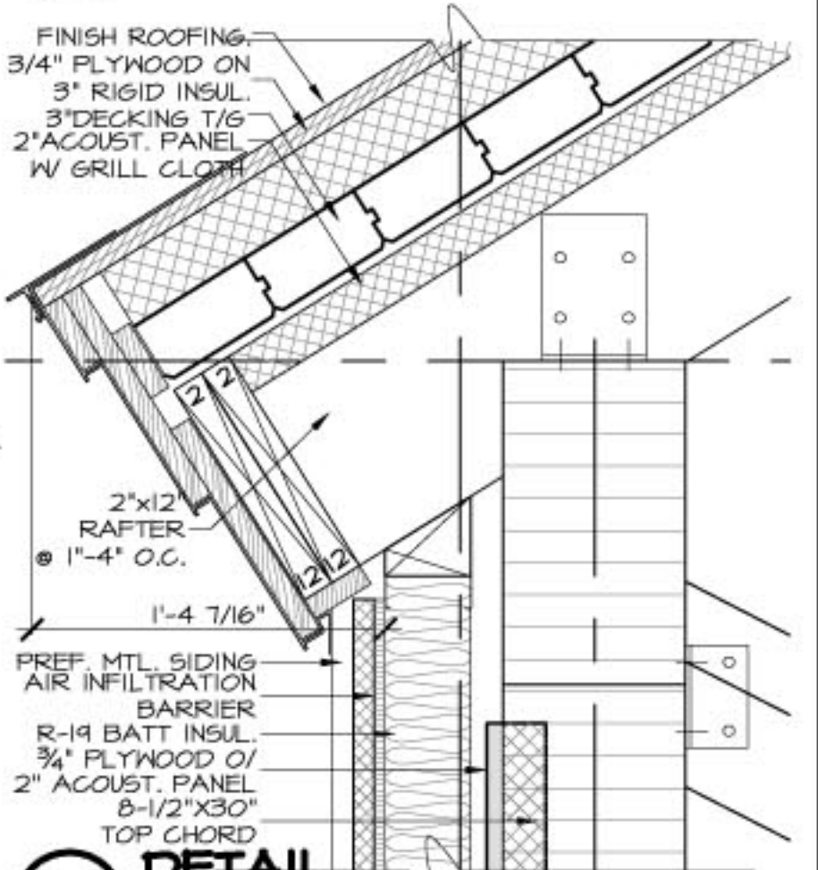
2.9 DETAIL SCALE: 1/2" = 1'-0"
