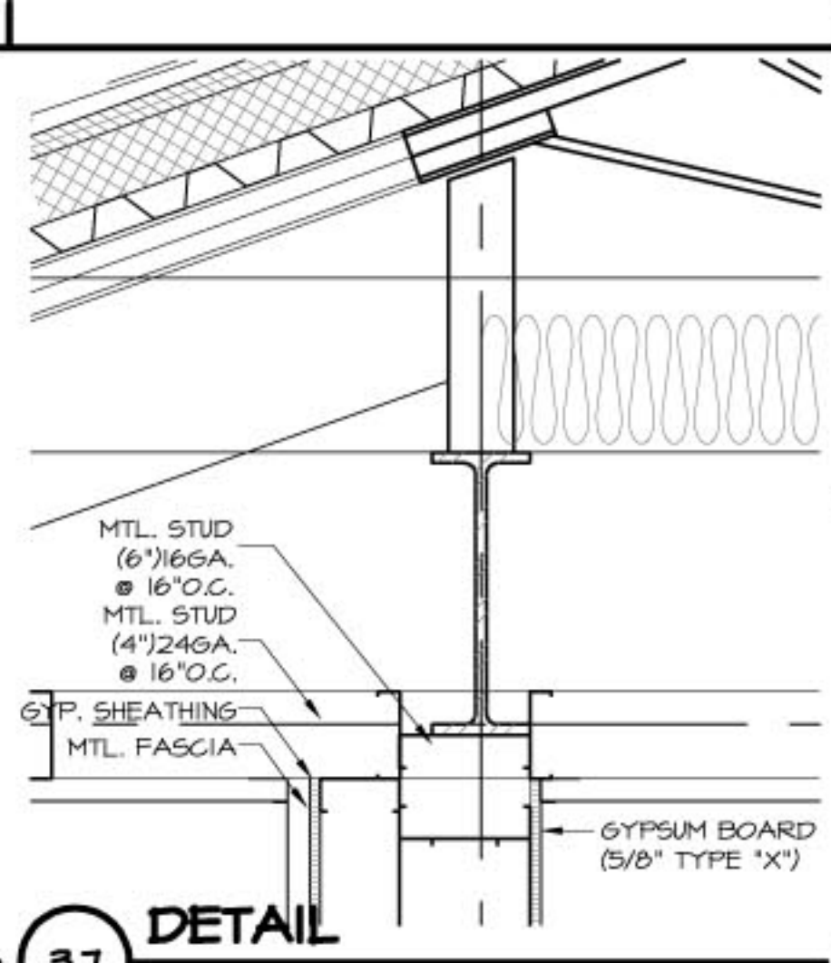
3.6 DETAIL SCALE: 1/2" = 1'-0"
