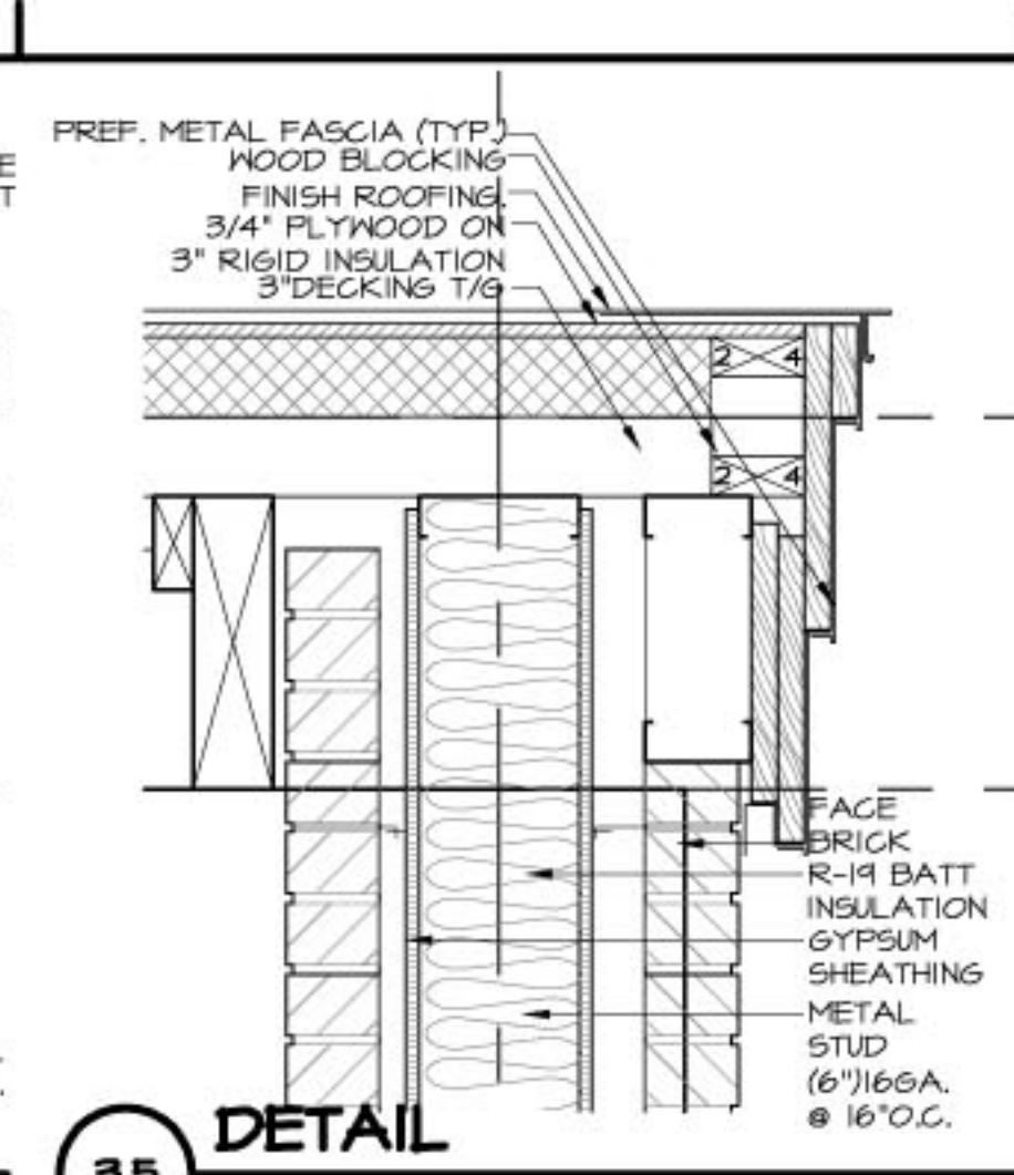
3.4 DETAIL SCALE: 1/2" = 1'-0"
