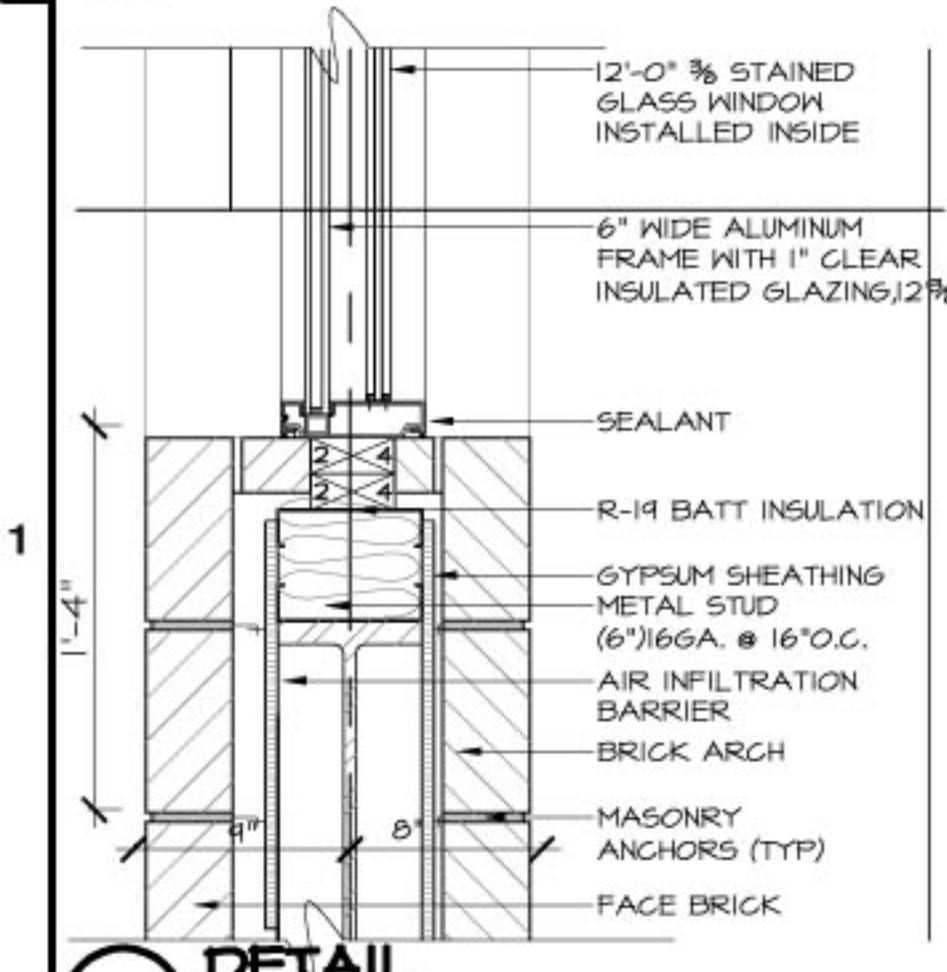
1.4 DETAIL SCALE: 1/2" = 1'-0"
