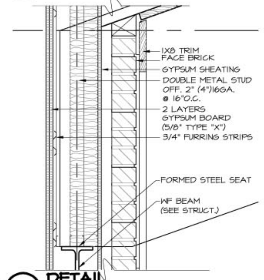
1.8 DETAIL SCALE: 1/2" = 1'-0"
