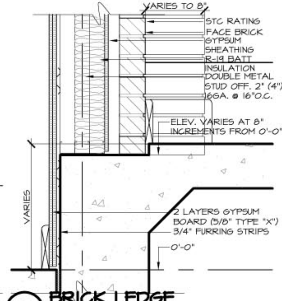
0.8 BRICK LEDGE SCALE: 1/2" = 1'-0"
