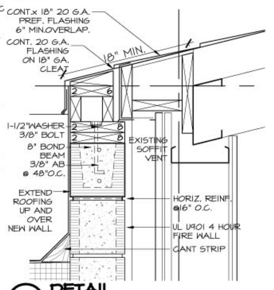
2.6 DETAIL SCALE: 1/2" = 1'-0"
