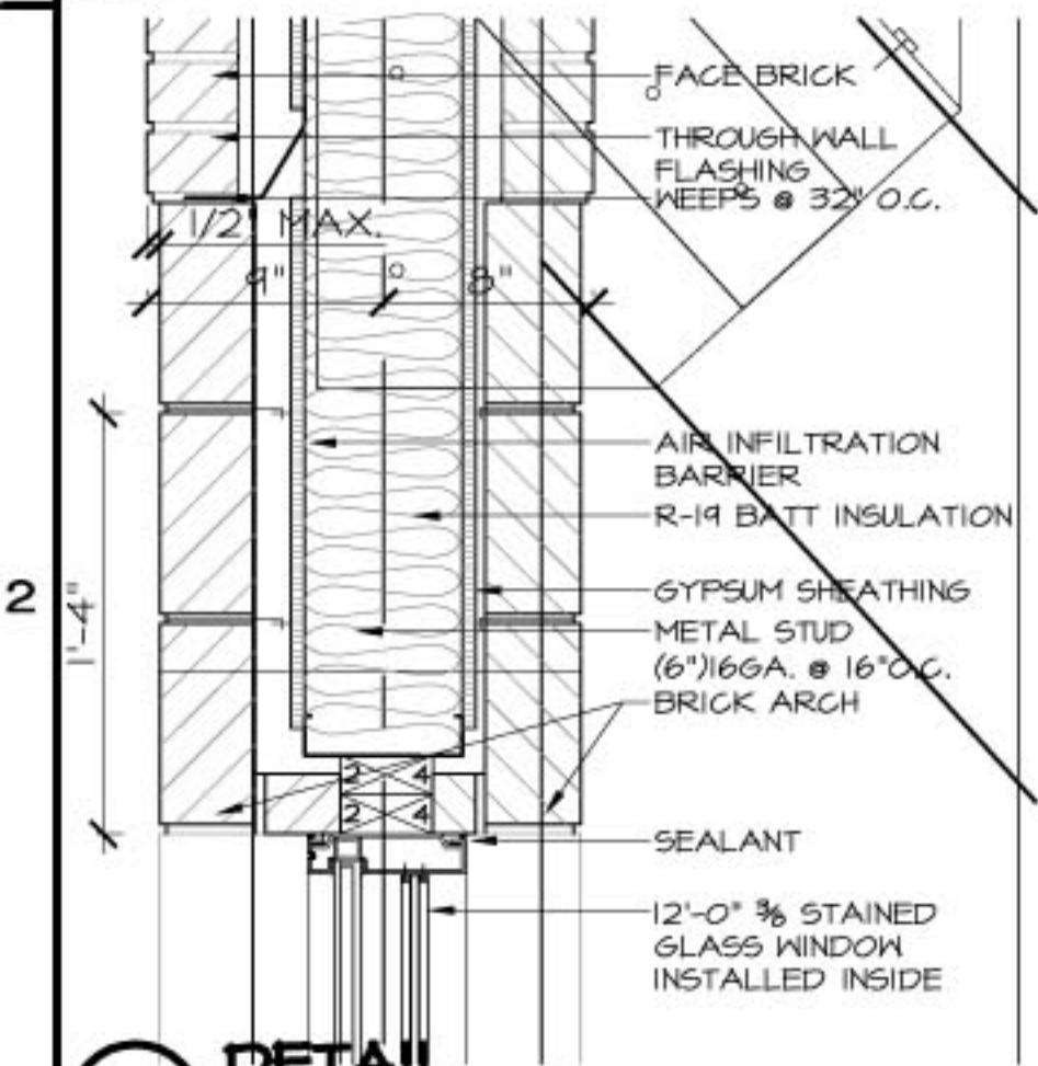
2.4 DETAIL SCALE: 1/2" = 1'-0"
