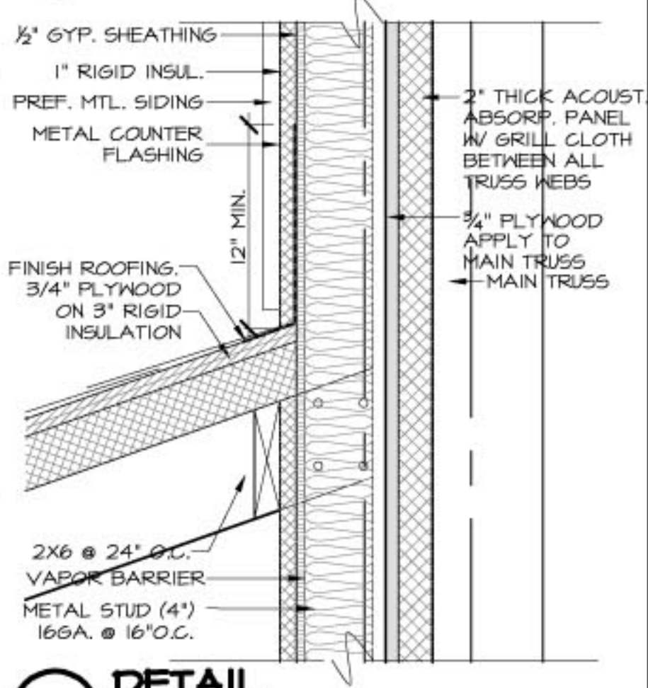
1.9 DETAIL SCALE: 1/2" = 1'-0"
