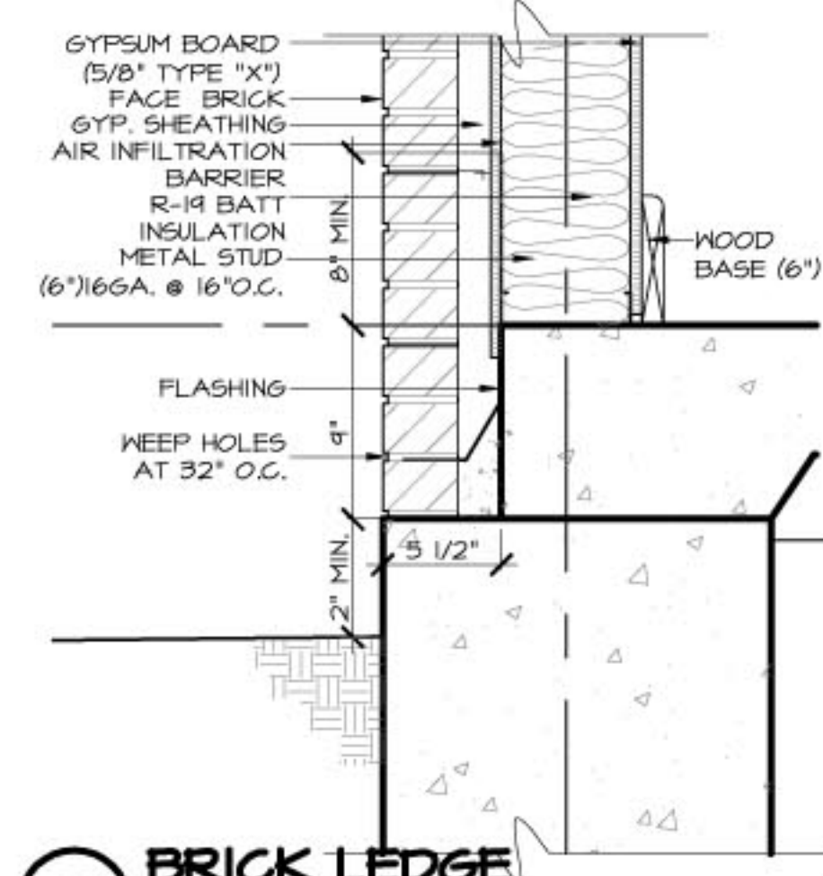
0.7 BRICK LEDGE SCALE: 1/2" = 1'-0"
