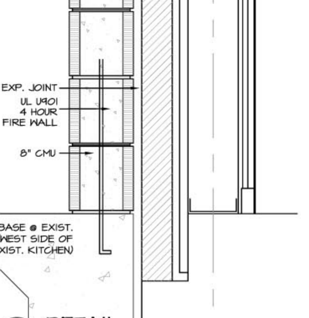
1.8 DETAIL SCALE: 1/2" = 1'-0"
