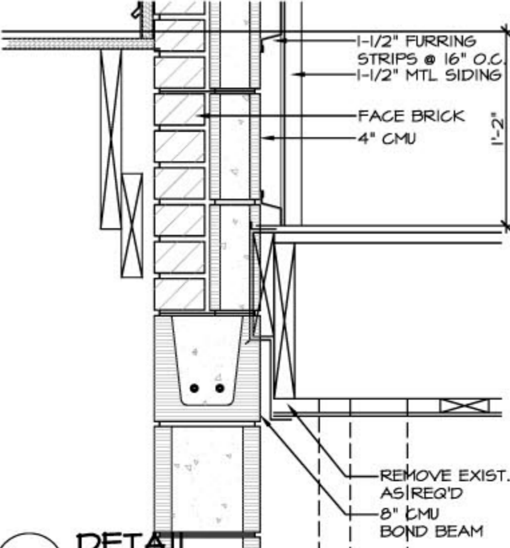
0.7 DETAIL SCALE: 1/2" = 1'-0"
