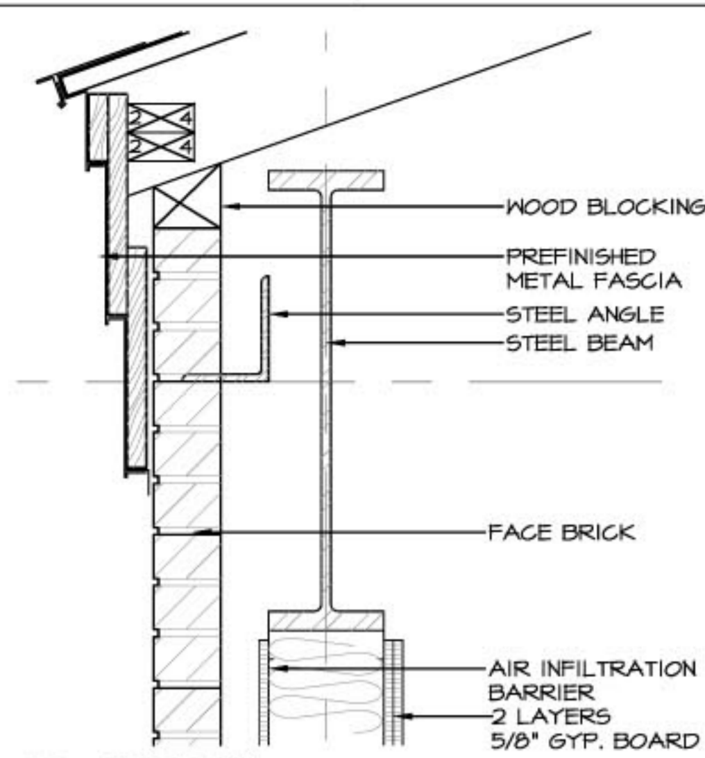
3.4 DETAIL SCALE: 1/2" = 1'-0"
