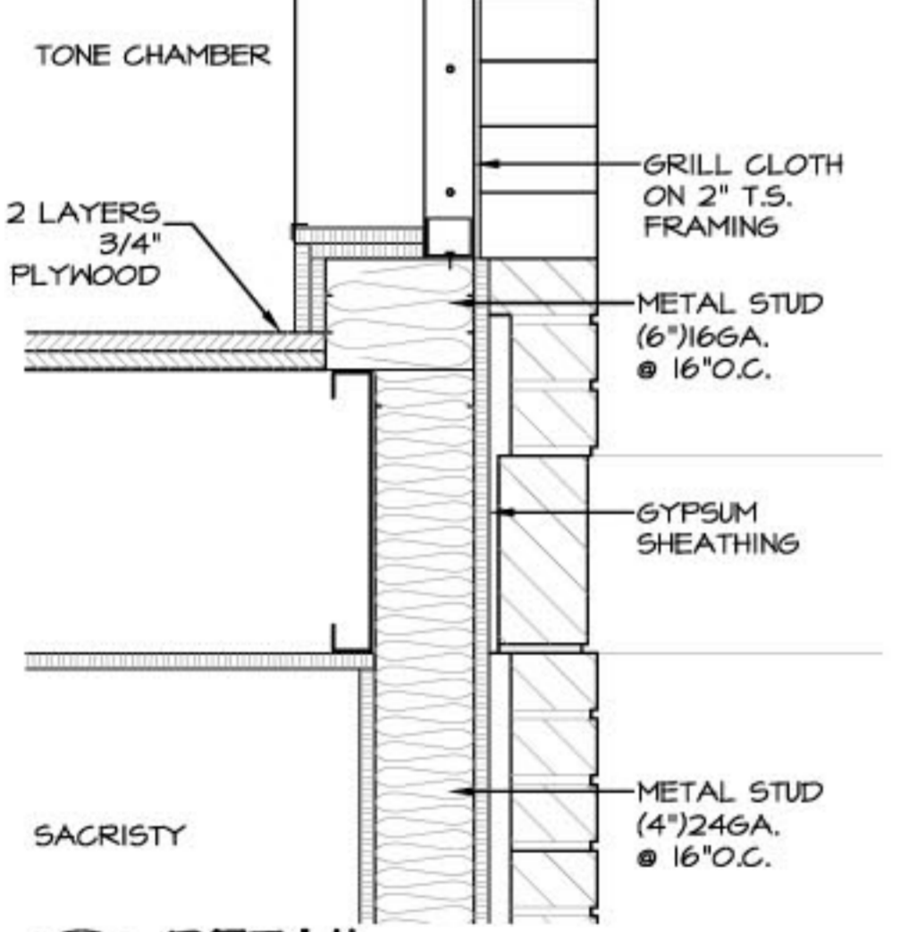
1.5 DETAIL SCALE: 1/2" = 1'-0"
