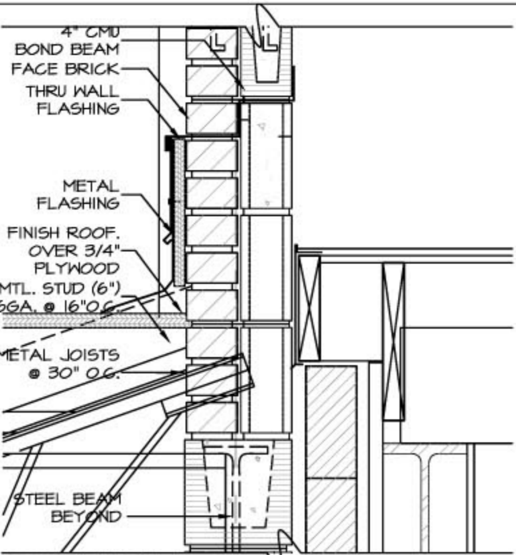
3.6 DETAIL SCALE: 1/2" = 1'-0"
