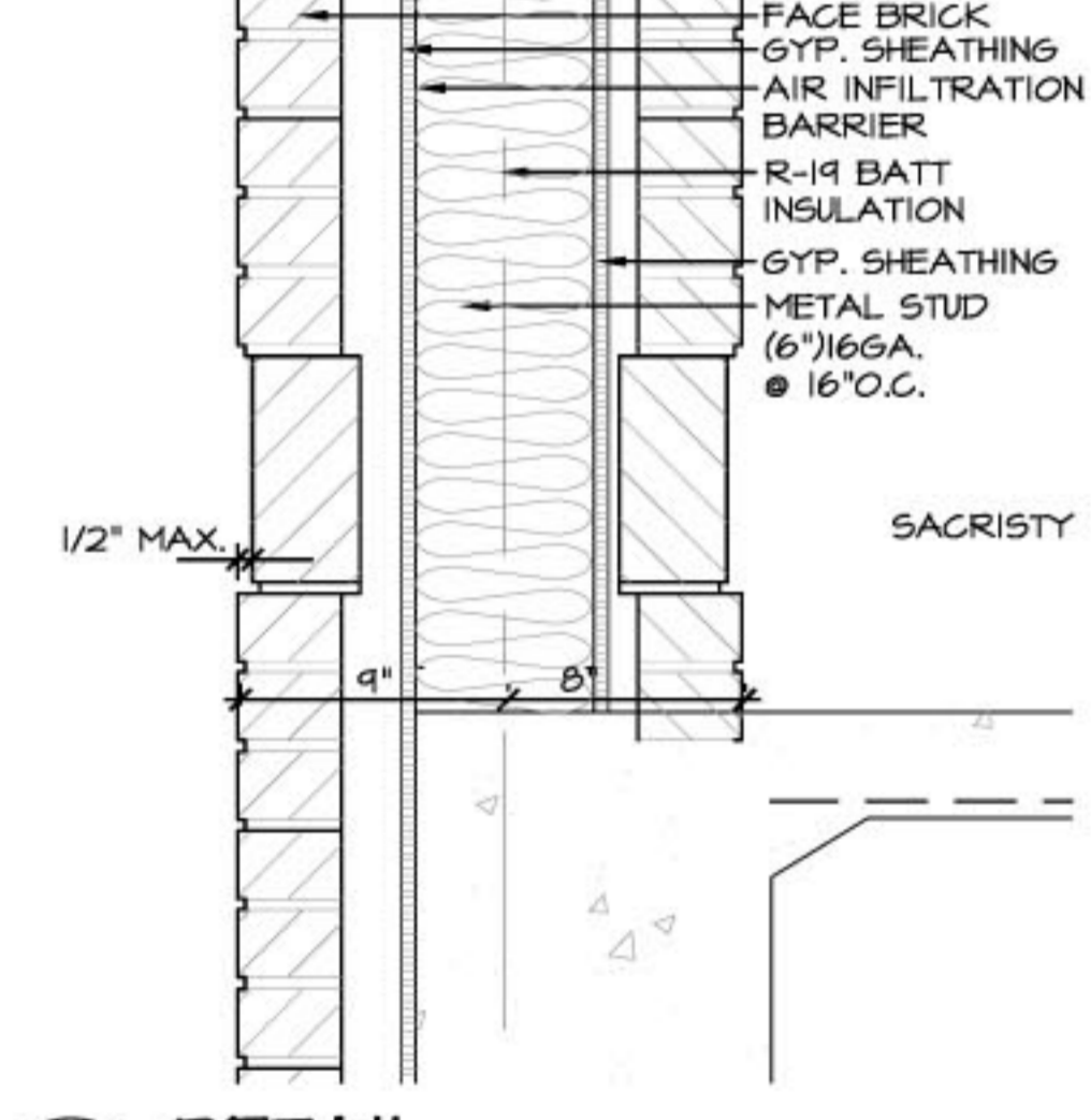
1.4 DETAIL SCALE: 1/2" = 1'-0"
