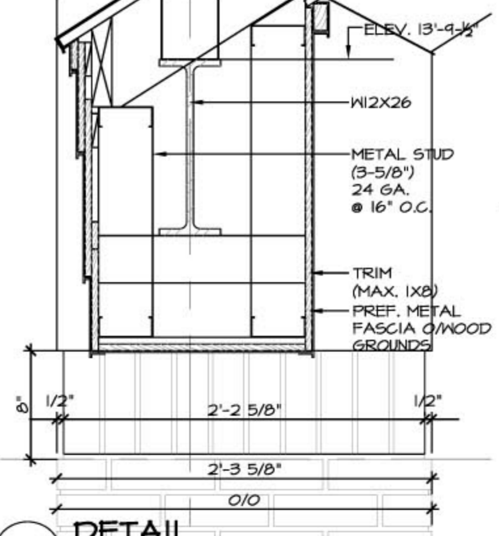
0.8 DETAIL SCALE: 1/2" = 1'-0"
