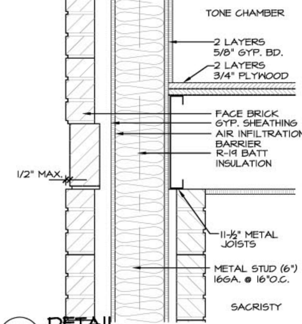
2.4 DETAIL SCALE: 1/2" = 1'-0"
