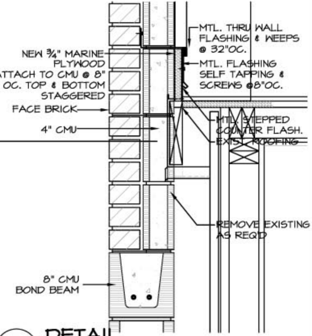
2.9 DETAIL SCALE: 1/2" = 1'-0"
