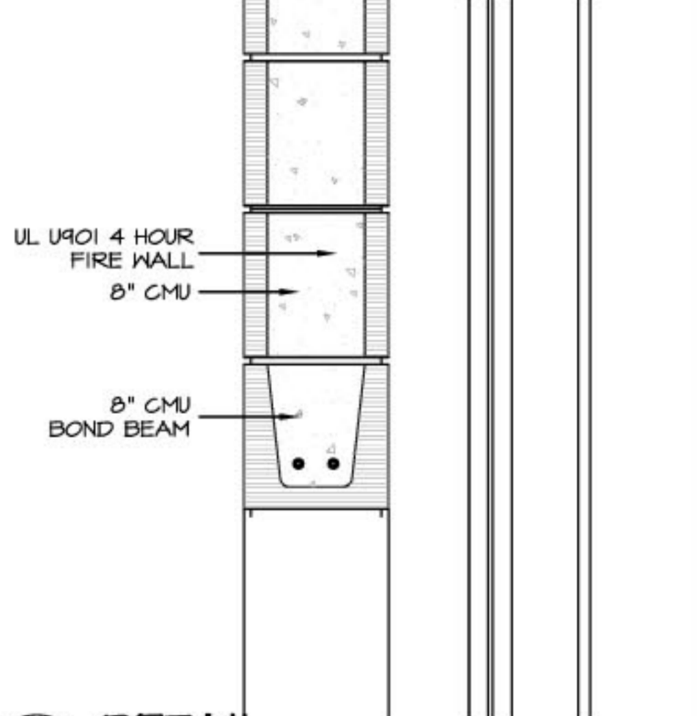
1.9 DETAIL SCALE: 1/2" = 1'-0"
