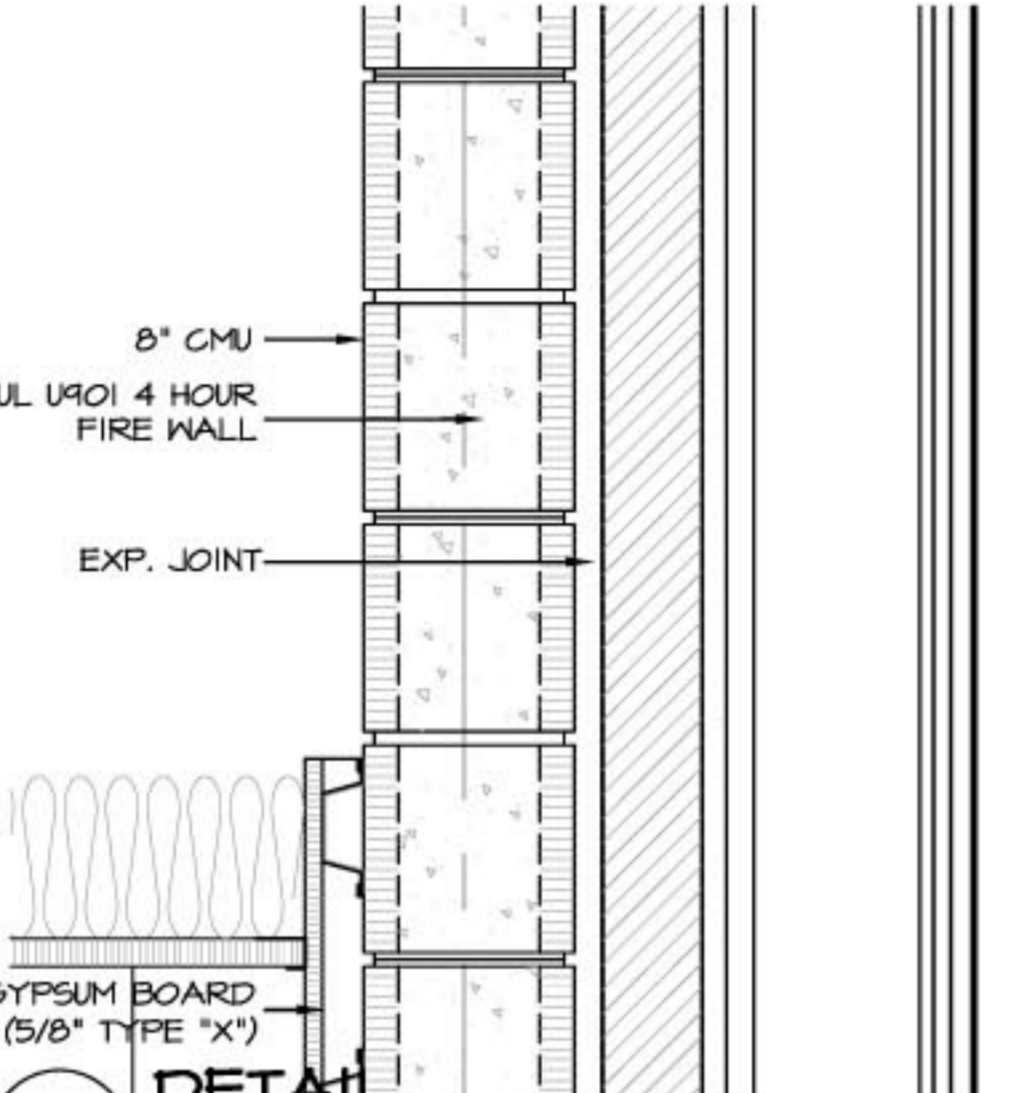
2.6 DETAIL SCALE: 1/2" = 1'-0"
