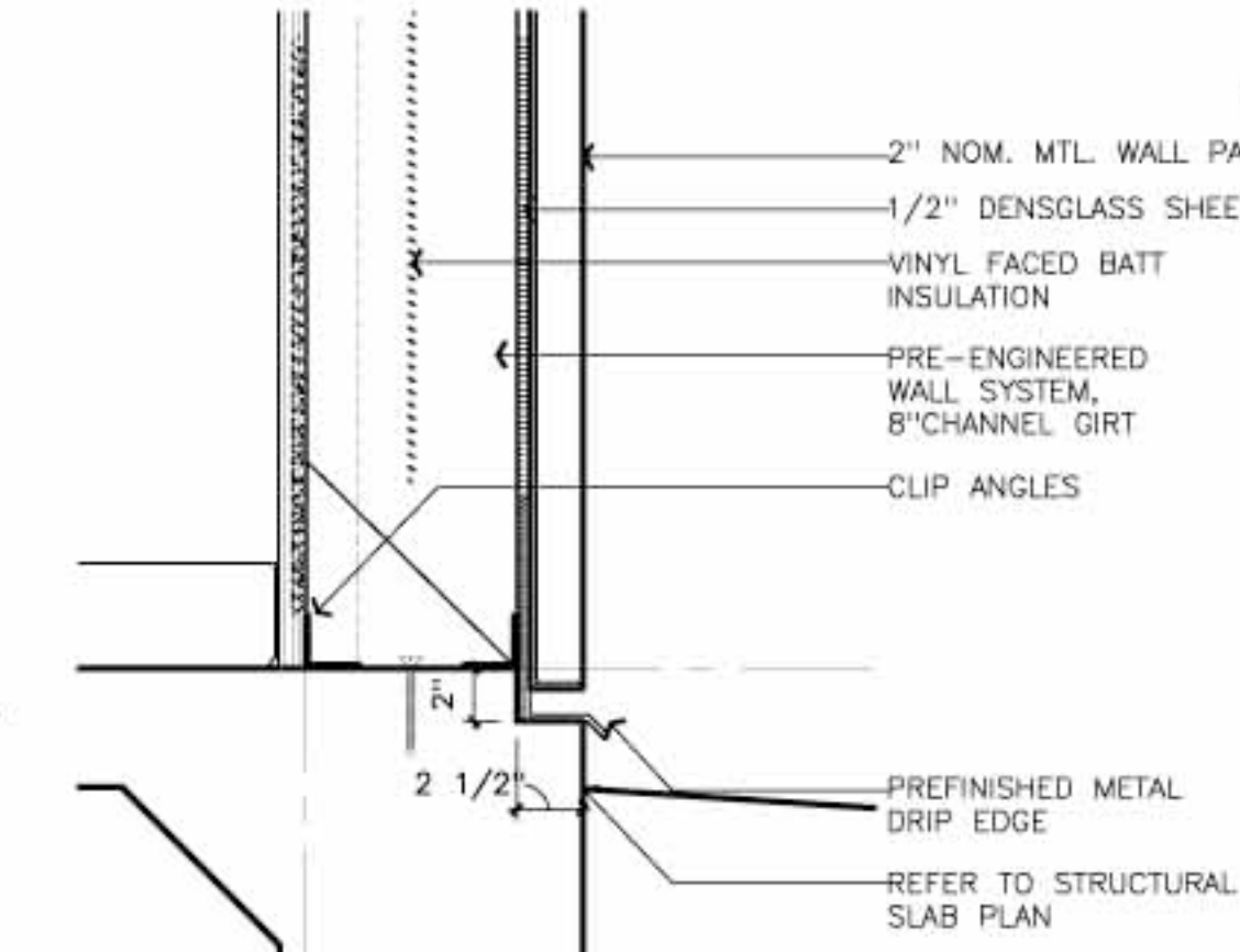
08 Detail SCALE: 1 1/2"=1'-0"
