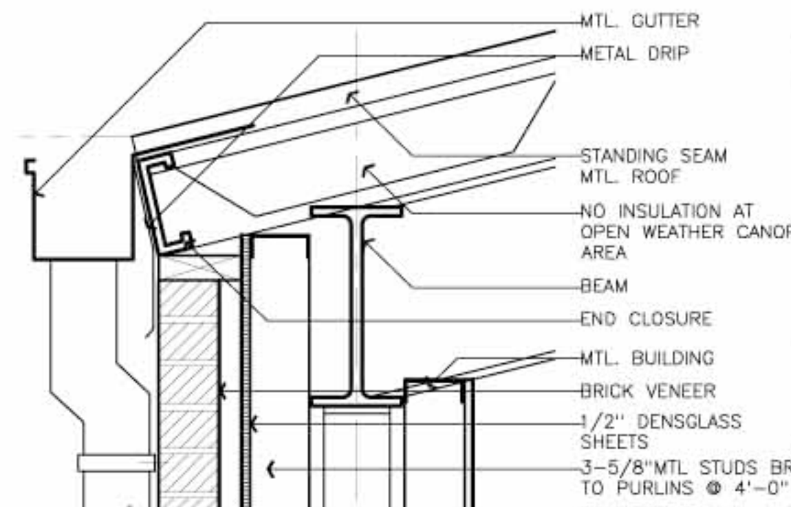
02 Detail SCALE: 1 1/2"=1'-0"
