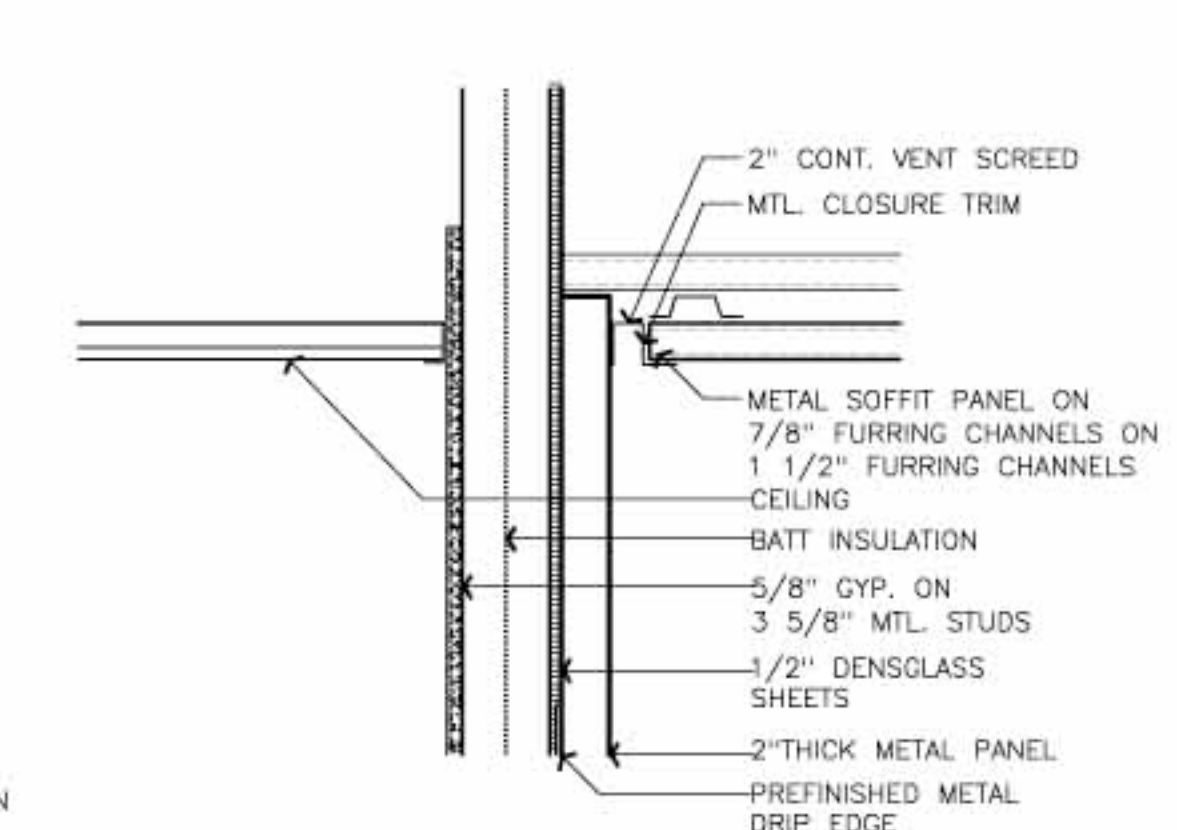
13 Detail SCALE: 1 1/2"=1'-0"
