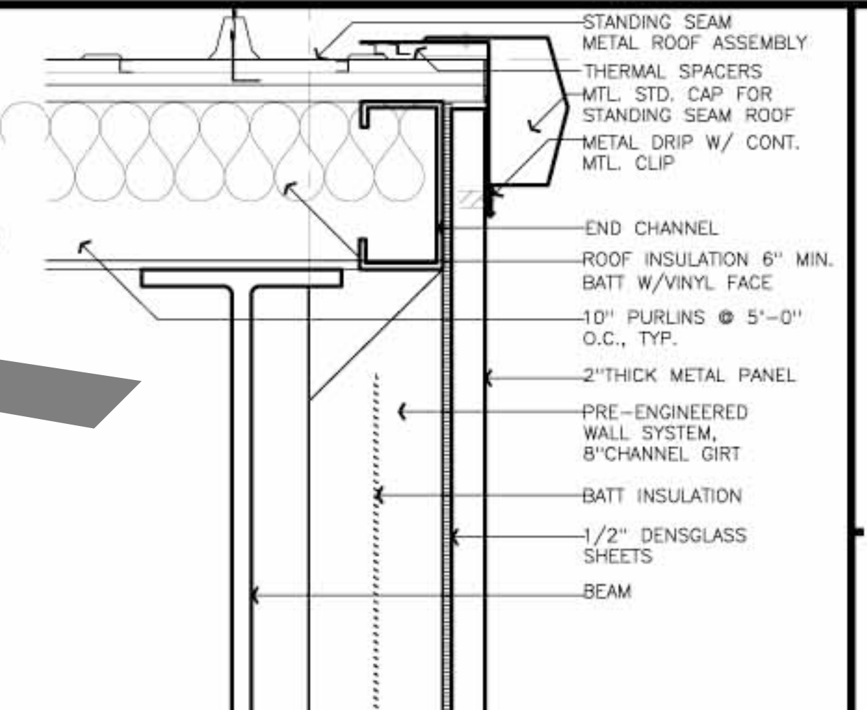
20 Detail SCALE: 1 1/2"=1'-0"
