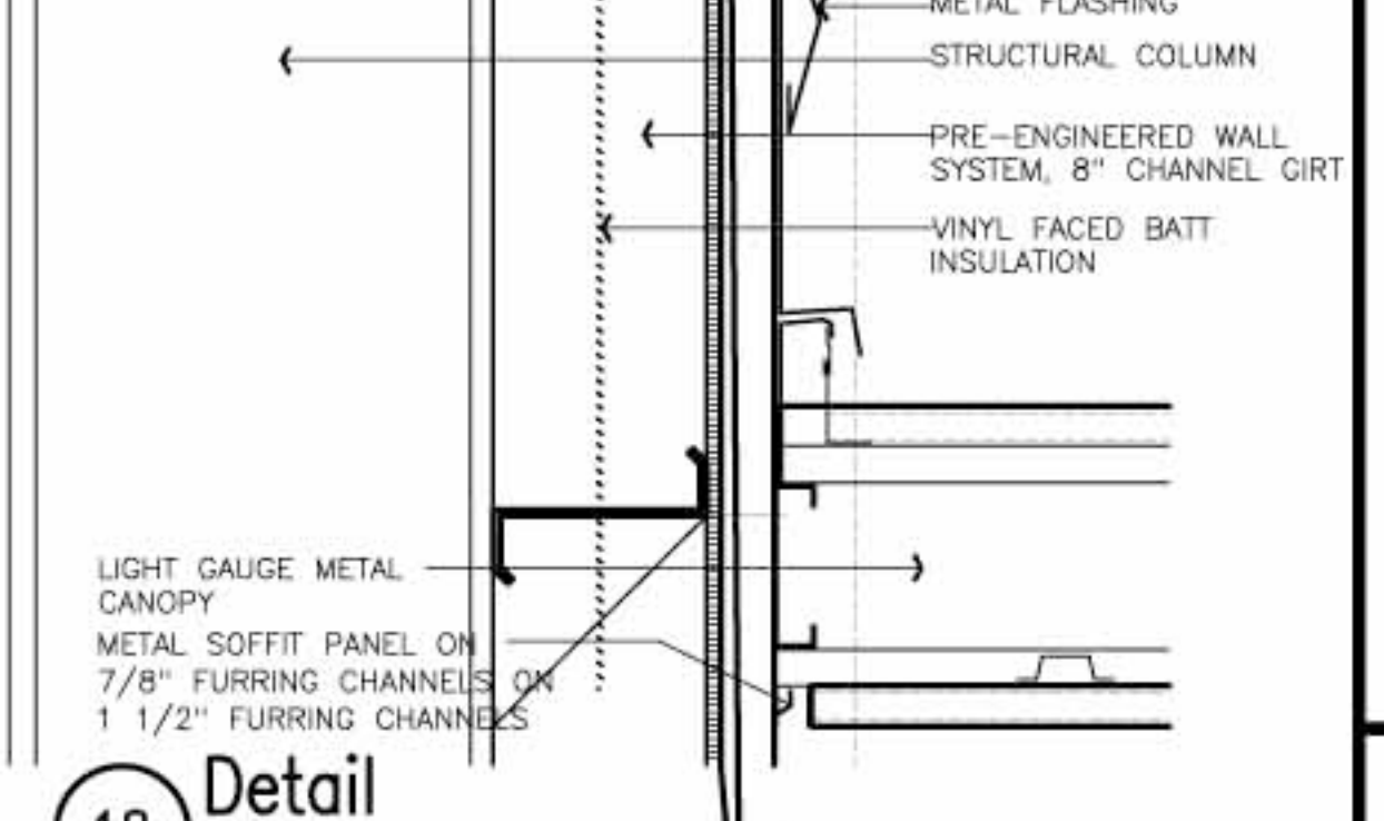
18 Detail SCALE: 1 1/2"=1'-0"
