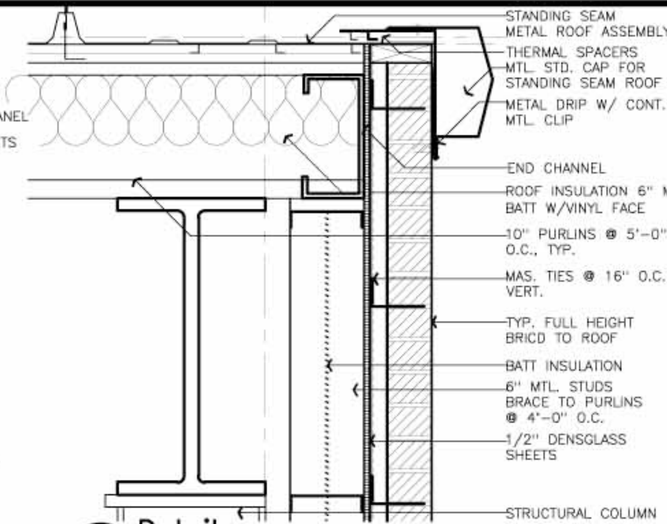
12 Detail SCALE: 1 1/2"=1'-0"
