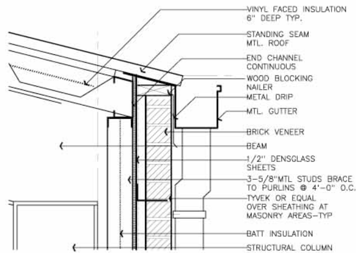
04 Detail SCALE: 1 1/2"=1'-0"
