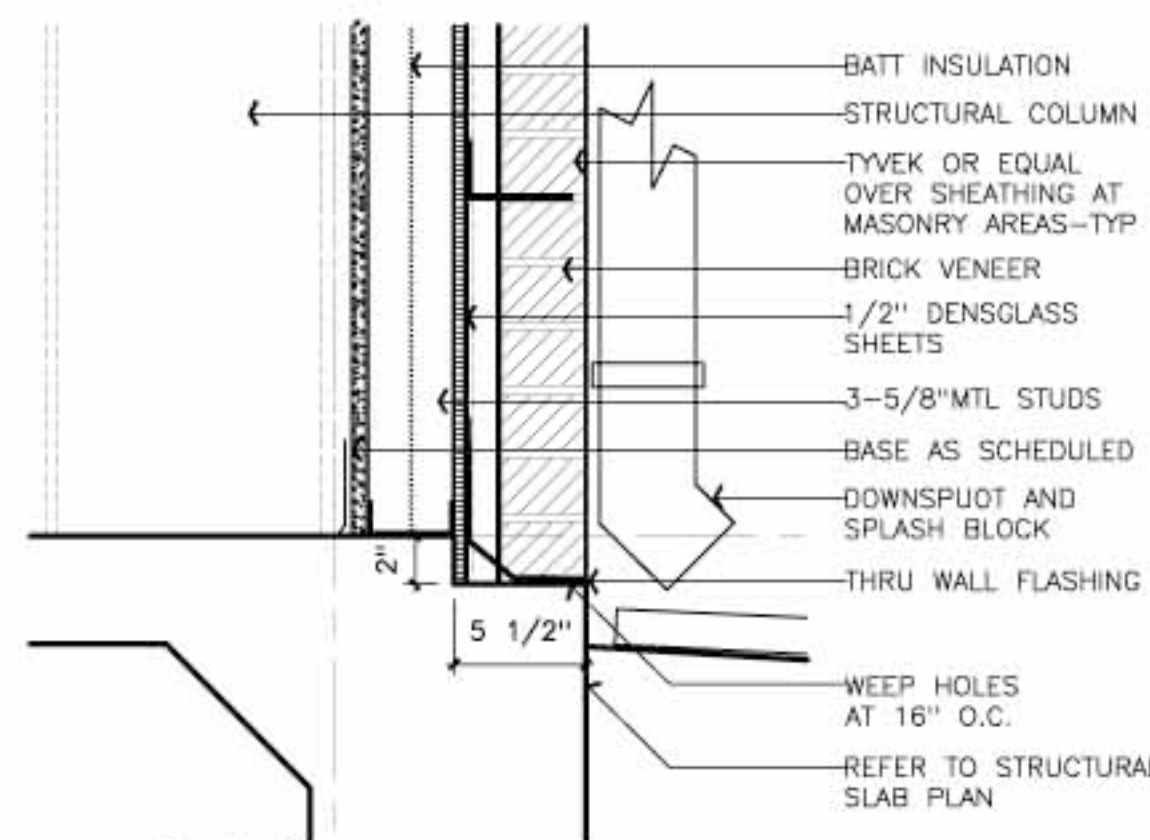
03 Detail SCALE: 1 1/2"=1'-0"
