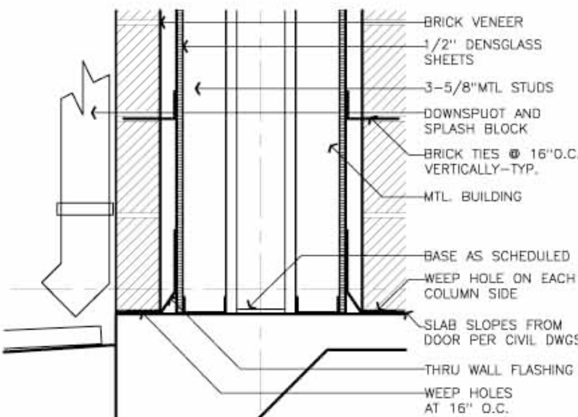
01 Detail SCALE: 1 1/2"=1'-0"
