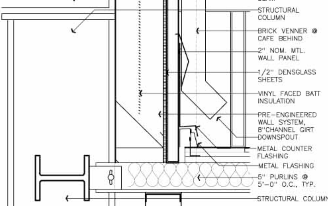
09 Detail SCALE: 1 1/2"=1'-0"
