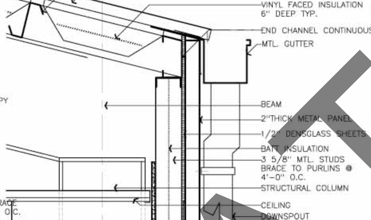
06 Detail SCALE: 1 1/2"=1'-0"
