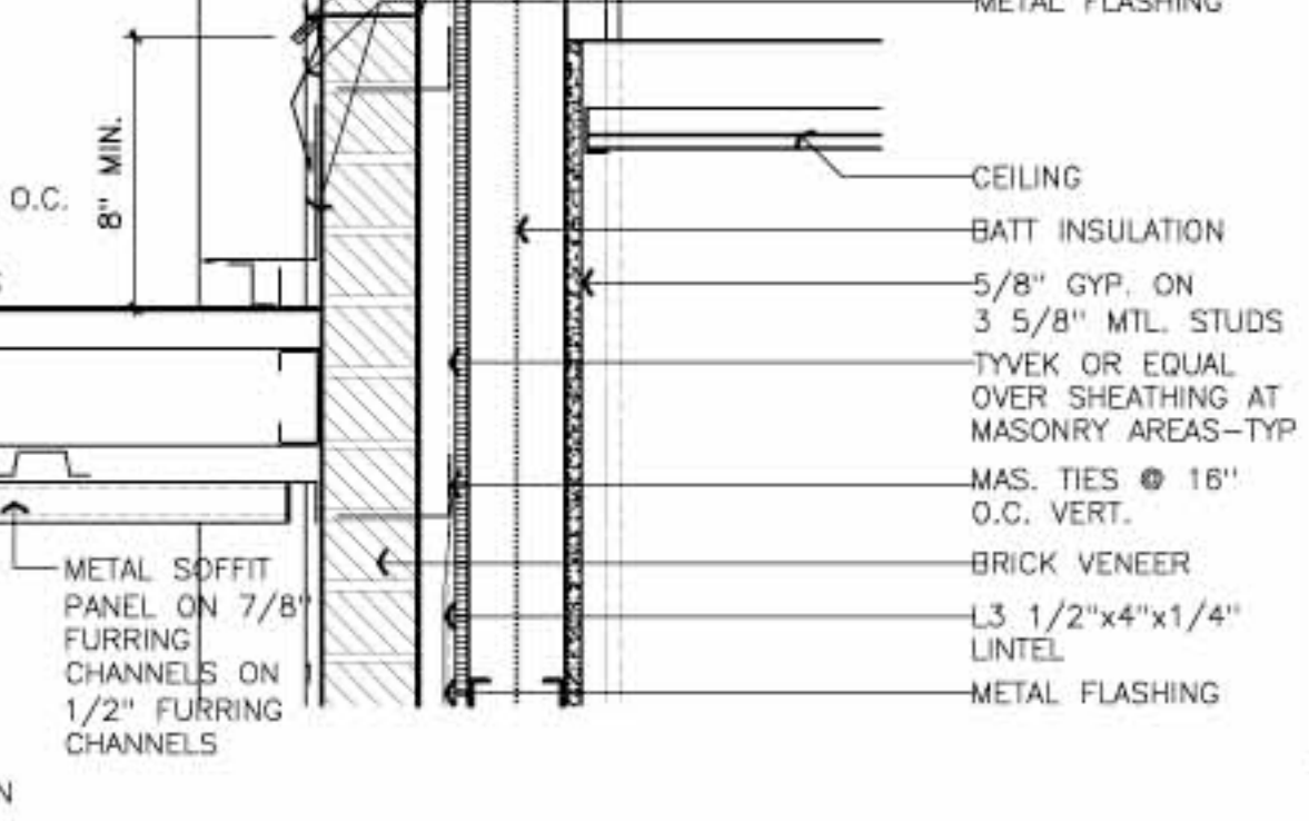
14 Detail SCALE: 1 1/2"=1'-0"
