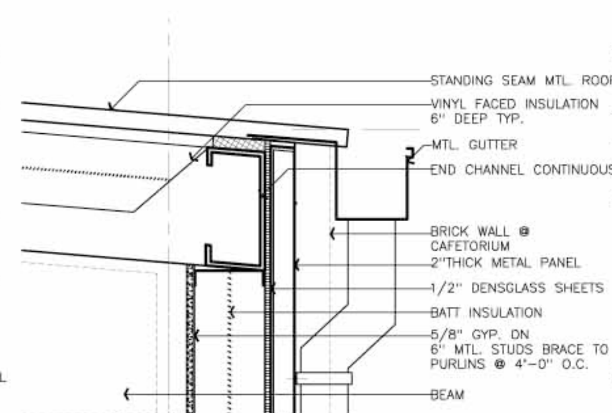
07 Detail SCALE: 1 1/2"=1'-0"
